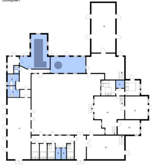
Stueplan
